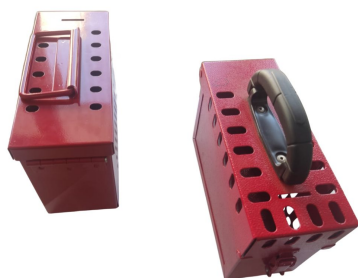
Caixa de Travamento 16 Ganchos — Fechada e Ventilada
