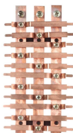
Barramento Trifásico Tipo Grade
