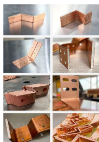
Barras Dobradas Formatos Variados
